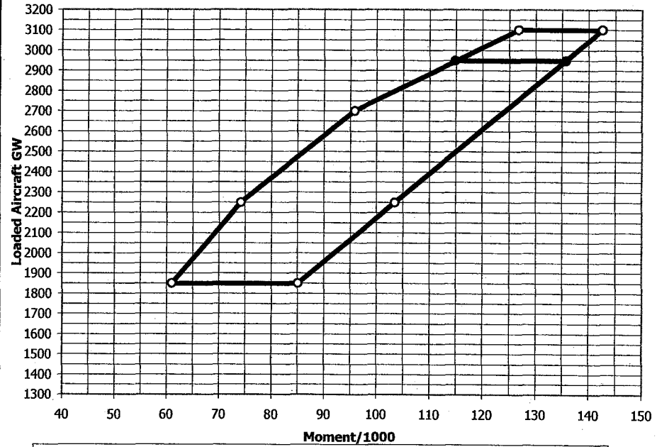
CG Moment Envelope
